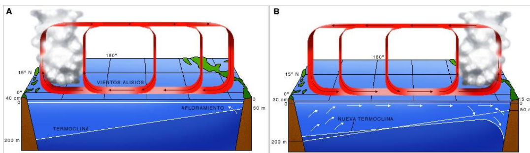
FIG.10 Circulación de vientos alisios en Pacífico Central y Oriental
