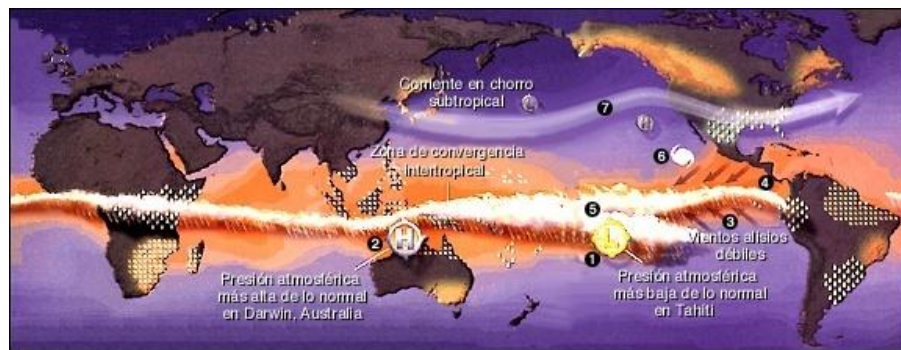
FIG.10 Circulación de vientos alisios en Pacífico Central y Oriental
